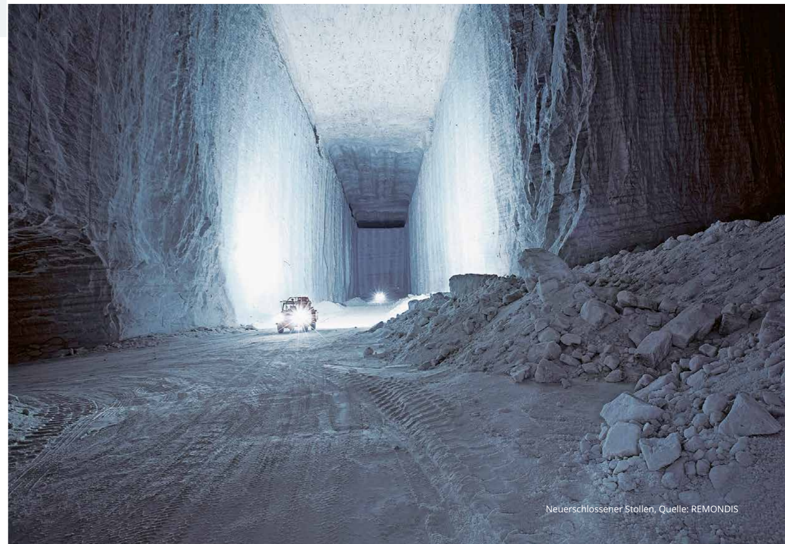
Bergmännische Technik im Untertageversatzbergwerk, Quelle: REMONDIS
